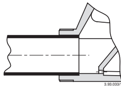
Abb. 1 Preßsitzverbindung.
